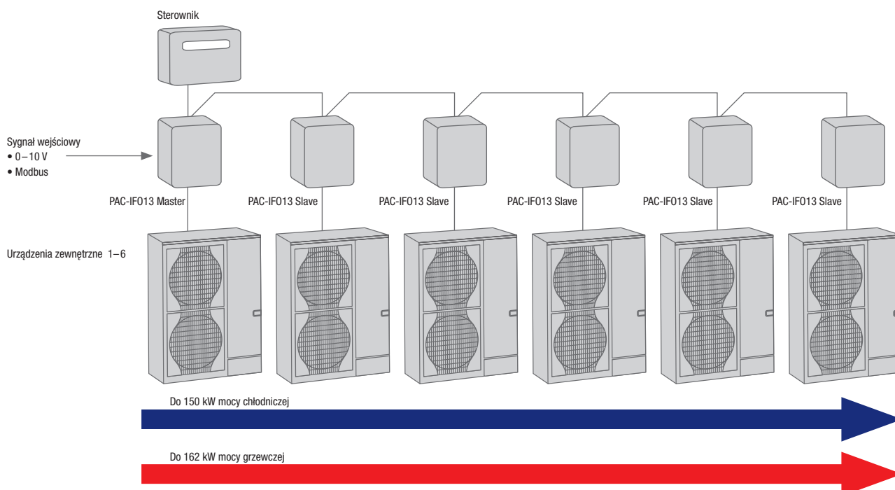
PAC-IF013B-E – moduł sterujący zewnętrznym wymiennikiem
