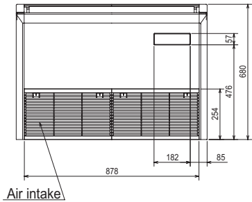
Urządzenia podstropowe PCA-RP35/50 KAQ
