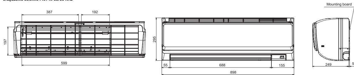
Urządzenia ściennie PKA-RP35/50 HAL
